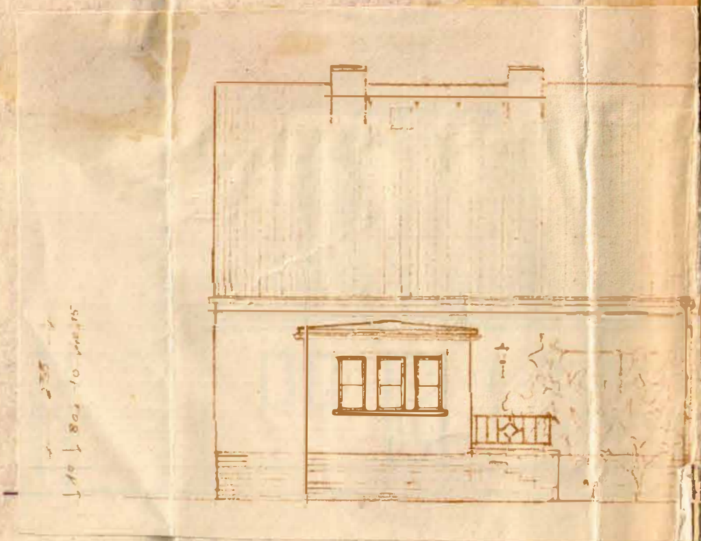
SEITENANSICHT
