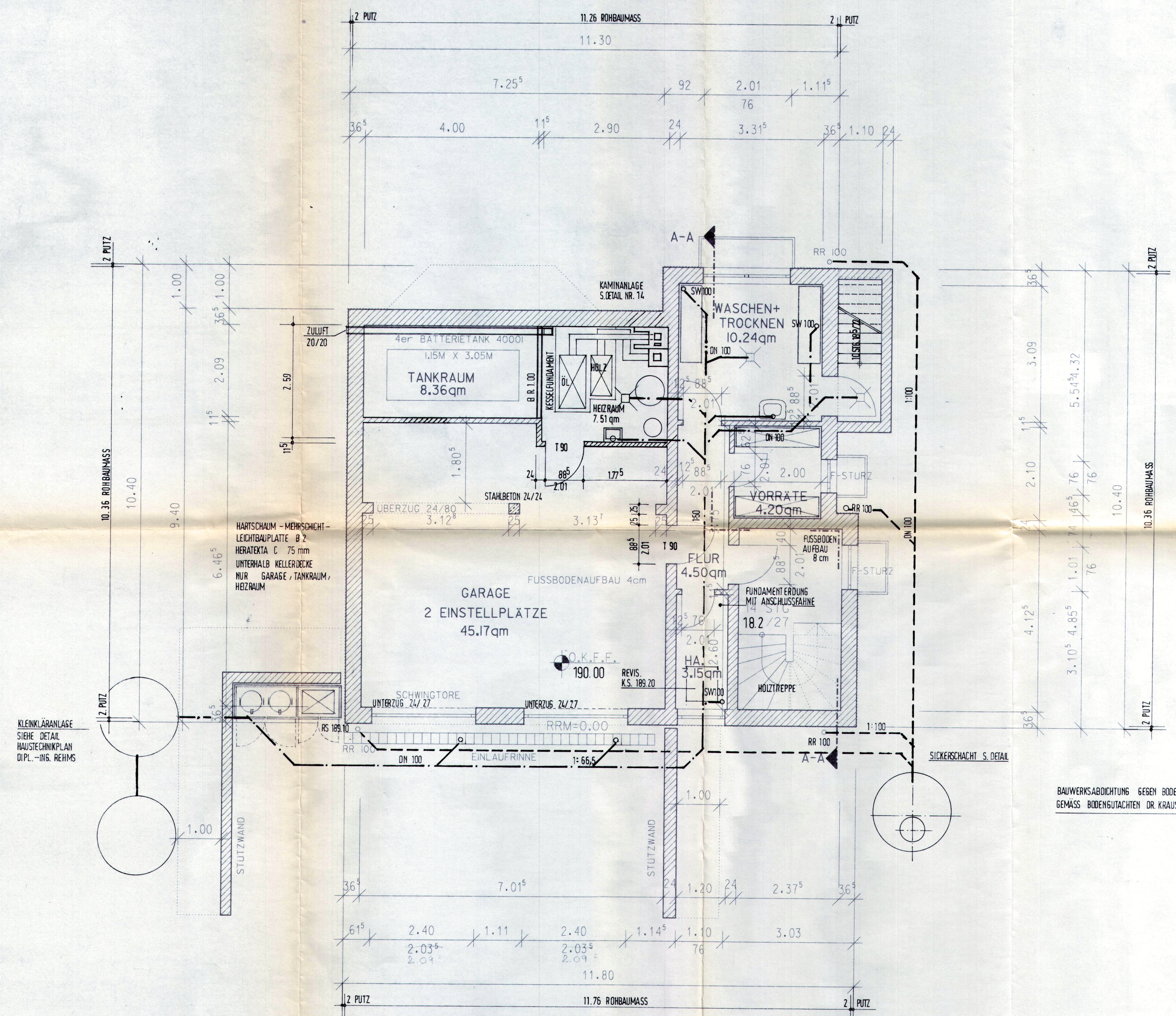
KELLERGECHOSS
